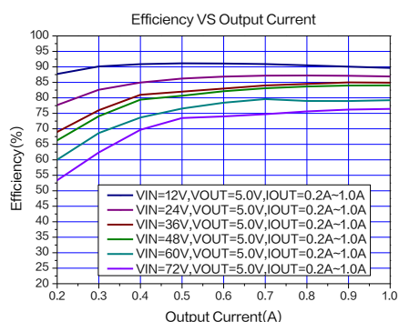
图1.XL9712典型应用示意图和转换效率曲线
