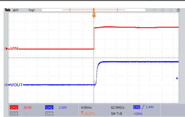
图 18.上电波形图 ( V_{IN}=48V , V_{OUT}=5.0V , I_{OUT}=0.1A )
