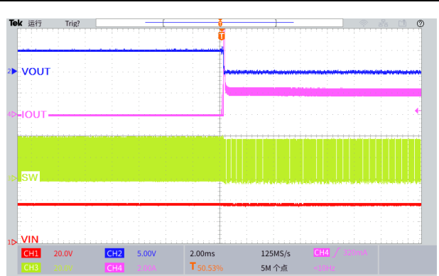
图 21.输出短路波形 ( V_{IN}=36V , V_{OUT}=5.0V )
