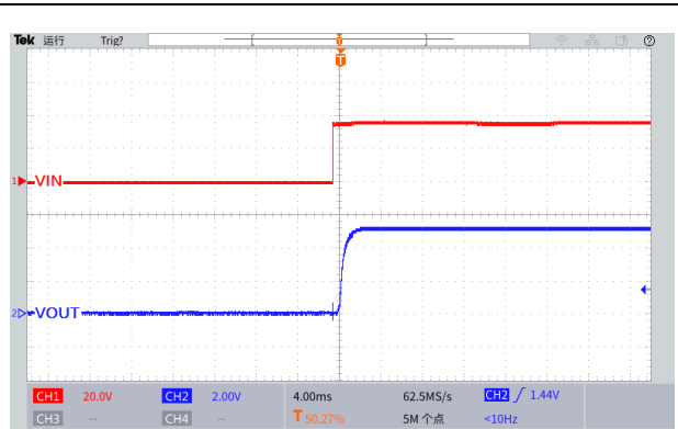
图 17.上电波形图 ( V_{IN}=36V , V_{OUT}=5.0V , I_{OUT}=0.1A )
