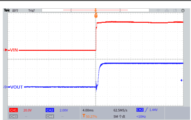
图 19.上电波形图 ( V_{IN}=60V , V_{OUT}=5.0V , I_{OUT}=0.1A )
