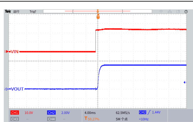
图 16.上电波形图 ( V_{IN}=24V , V_{OUT}=5.0V , I_{OUT}=0.1A )
