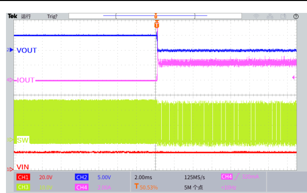
图 20.输出短路波形 ( V_{IN}=24V , V_{OUT}=5.0V )
