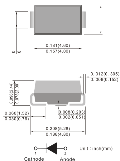
SMA/DO-214AC
