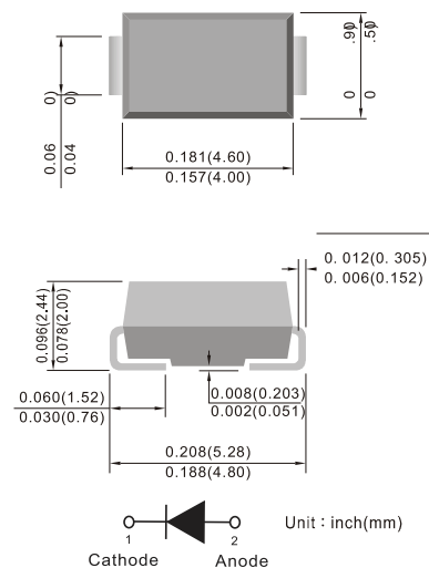
SMA/DO-214AC
