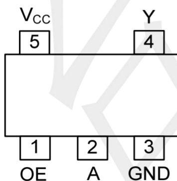
SOT23-5 / SOT353
