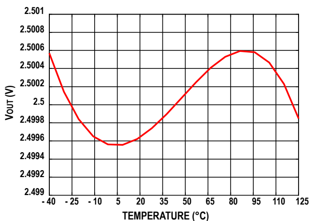
图4. ADR4525 典型输出电压与温度关系
