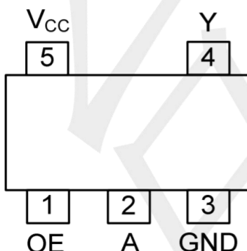
SOT23-5 / SOT353
