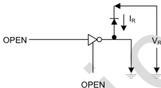
6. I_R
