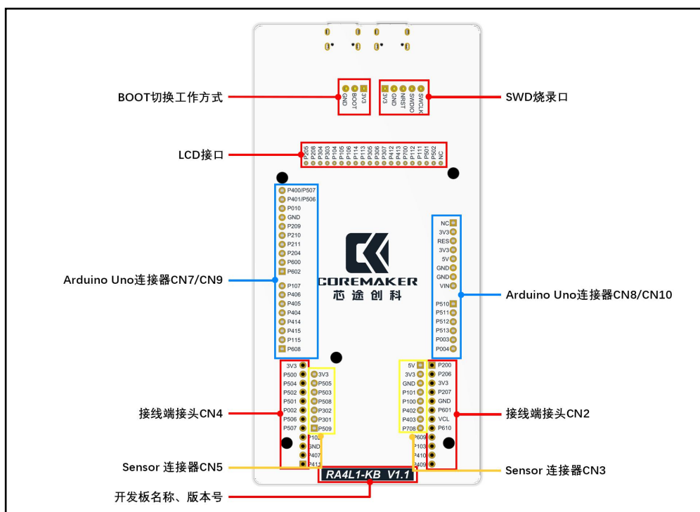
图 2 RA4L1 & KB 开发板（背面）
