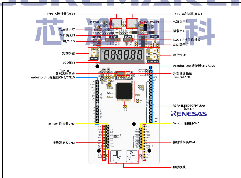
图 1 RA4L1 & SENSOR 开发板 (正面)
