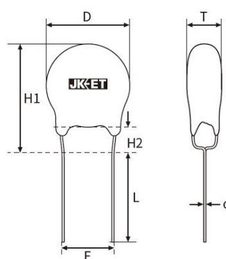
类型 D: Y 形脚
