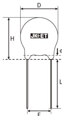
类型 A: 直脚
