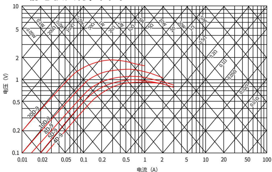
XXD-9电压-电流曲线
