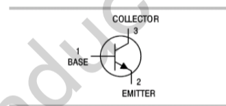
SOT-23
