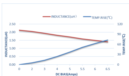
ZETC303015D-2R2MT-LF
