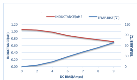
ZETC303015D-1R0MT-LF
