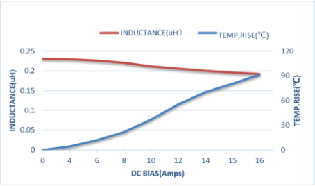
ZET-CORE-303018DTR22MBCA
