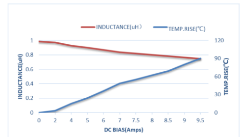
ZETC404012S1R0MBT-LF
