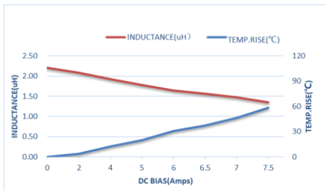
ZET-CORE-404012ST2R2MBCA
