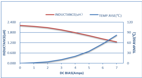
ZEP1M303012D-2R2M
