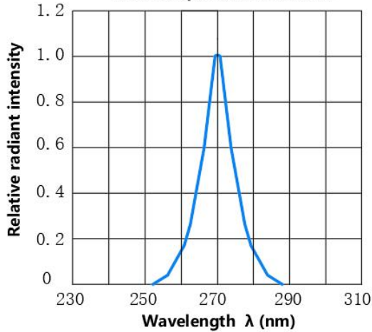
光谱分布曲线 Relative Spectral Distribution
