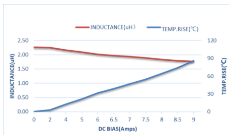
ZEMS404020-2R2M
