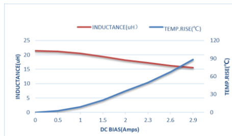
ZEMS404020-220M
