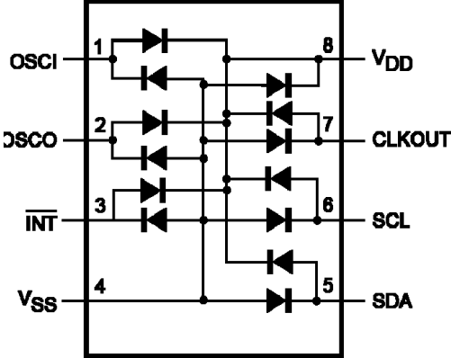
管脚二极管保护图:
