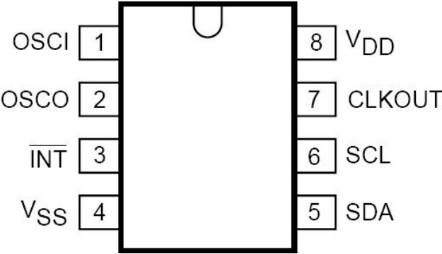
管脚排列图:
