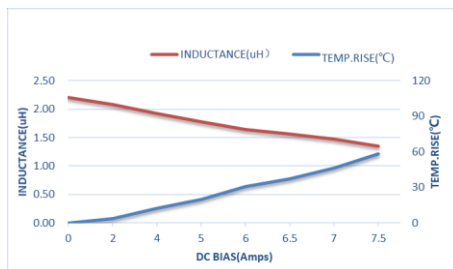
ZET-CORE-404012ST2R2MBCA
