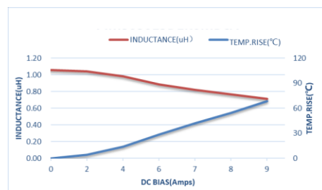
ZEMS303015-1R0M
