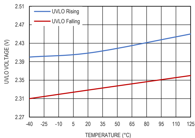
图 13. UVLO 阈值
