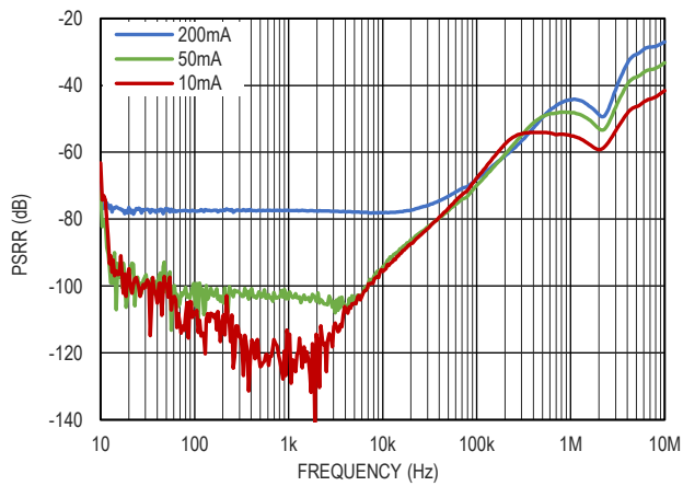
图 18. 电源电压纹波抑制比, V_{IN}=4.1V , V_{OUT}=3.6V
