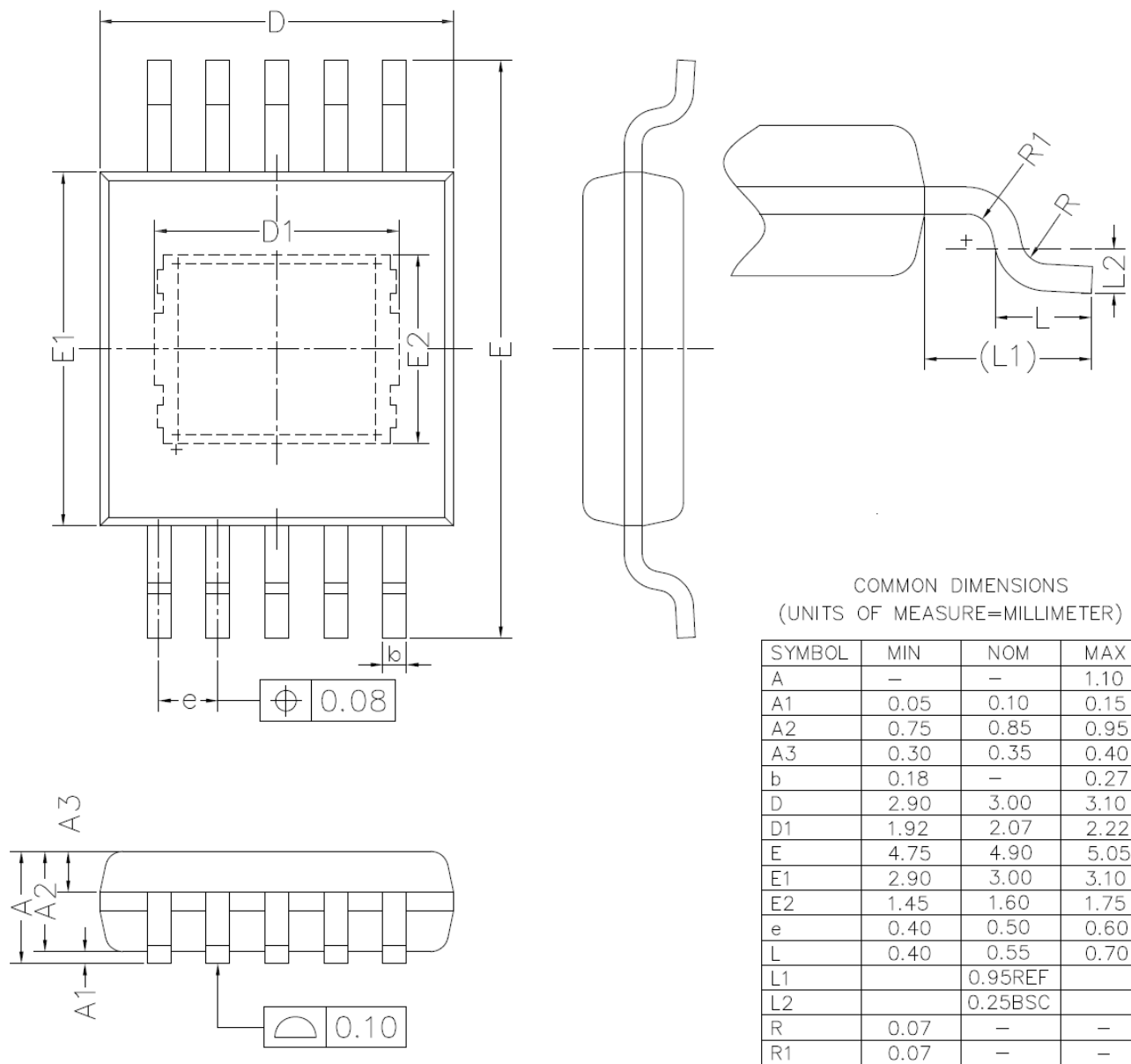
图 24 MSOP 封装
