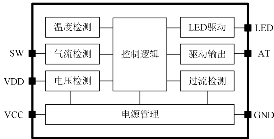
图 9-1 NSL2020B 功能框图
