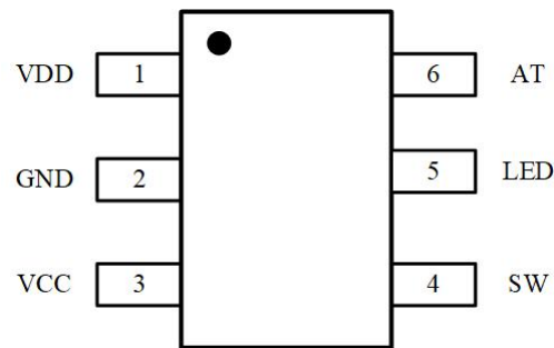
图 6-1 6-脚 SOT 顶视图
