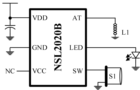
图 9-2 典型应用电路图 1
