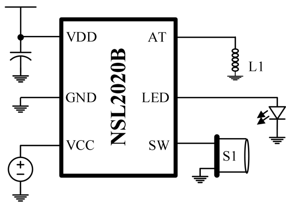
图 9-3 典型应用电路图 2
