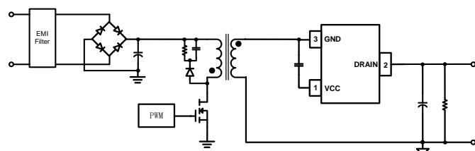
High SR 浮地应用
