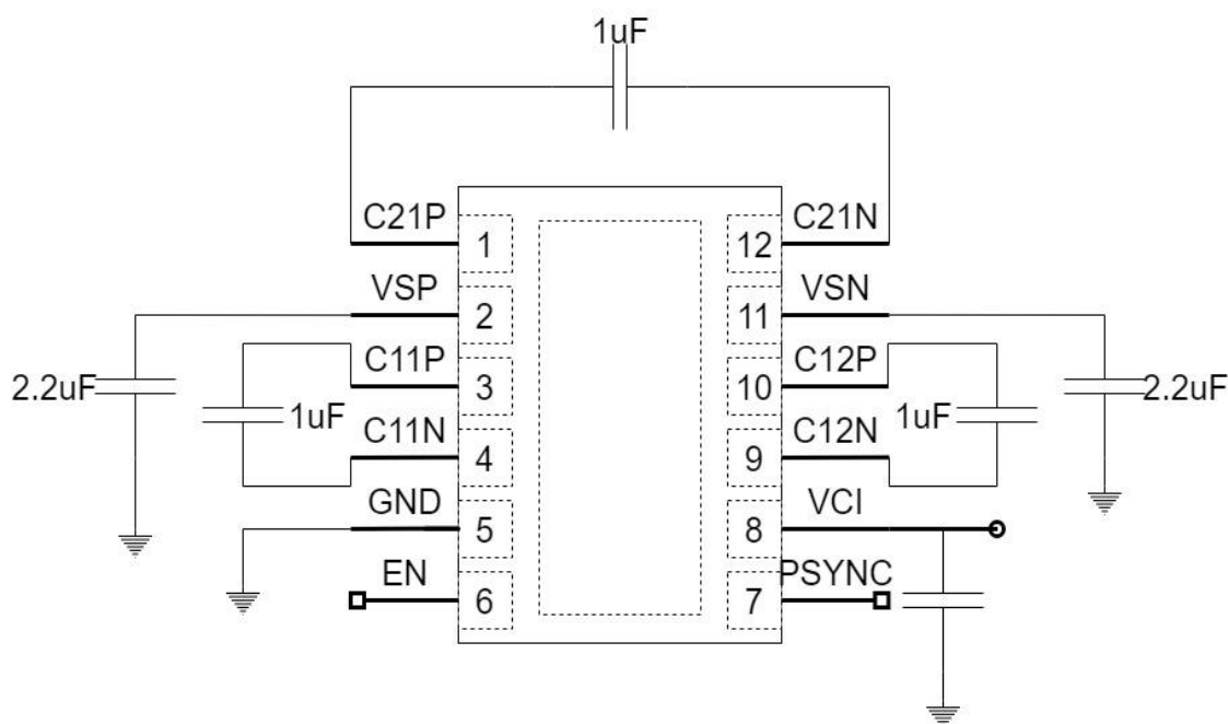
图 1.FDT7721 典型应用图
