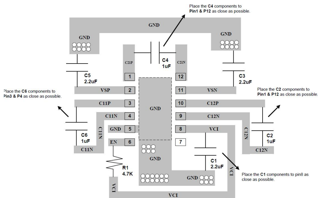
图 5. 布局参考图
