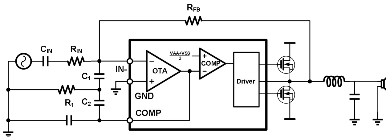
图 10-3 NSA20921 典型控制环路设计
