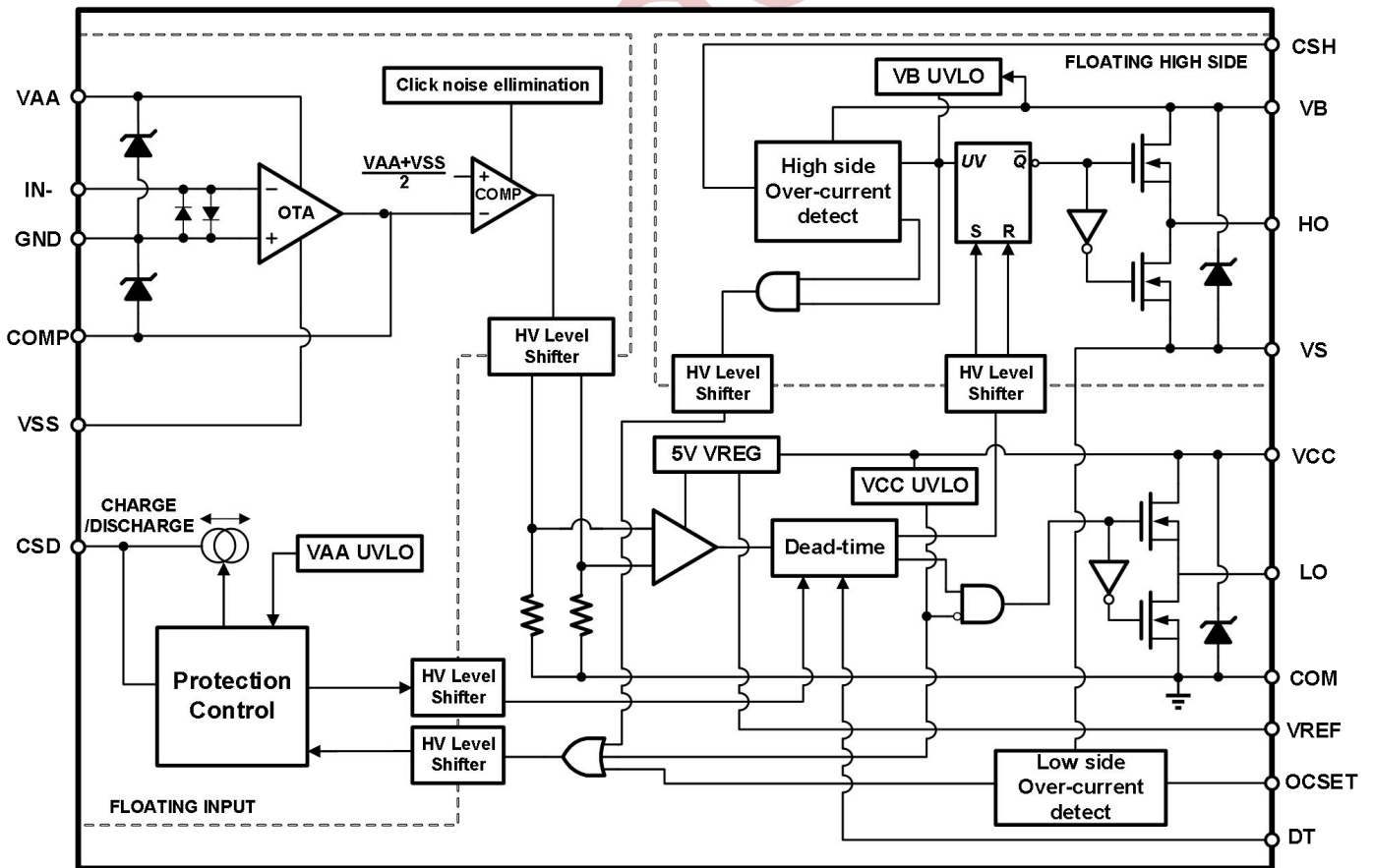
图 10-1 全芯片功能框图
