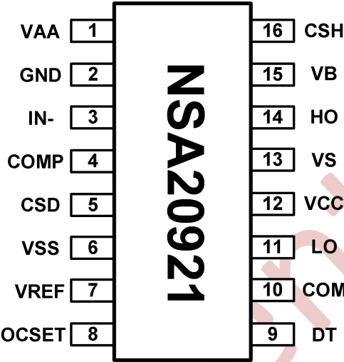
图 6-1 16-脚 SOP 顶视图
