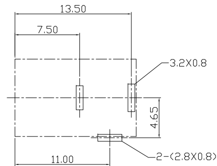
P.C.B 设计参考尺寸
