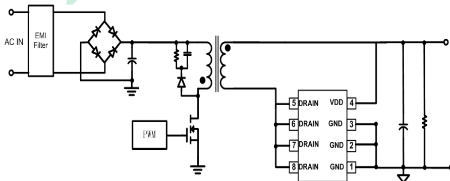
Low Side 实地应用 (5V 系统无需 VDD 电容)
