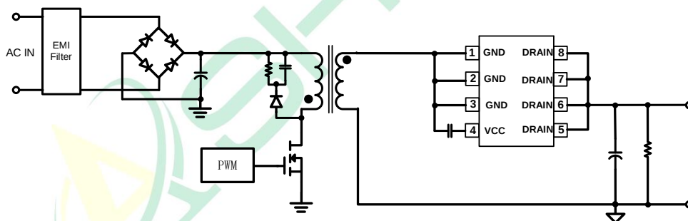
High SR 浮地应用
