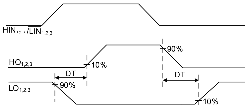
图 9-3 延时匹配波形定义
