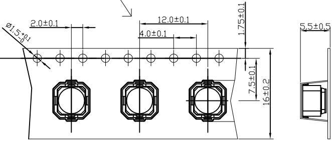
图2 成品盘带
