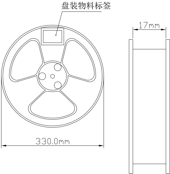
图3 盘装料盘
