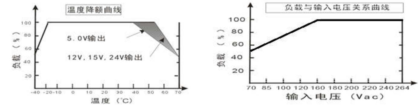
降额曲线图
