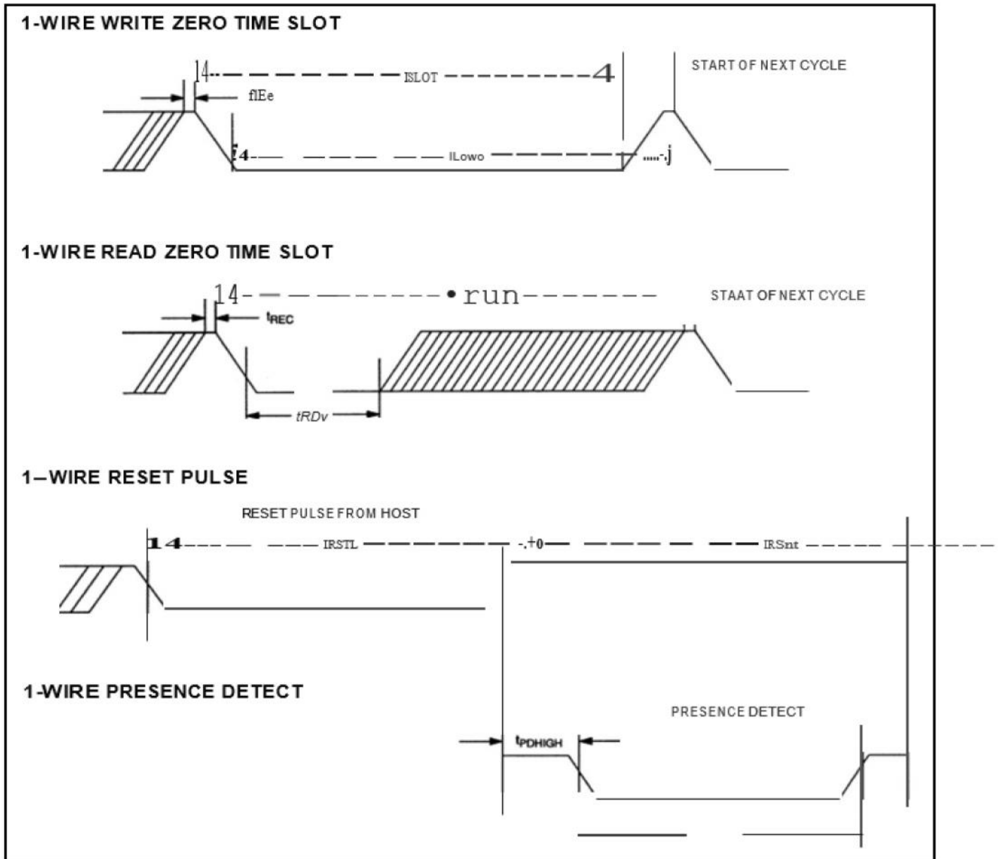
图 18. 时序
