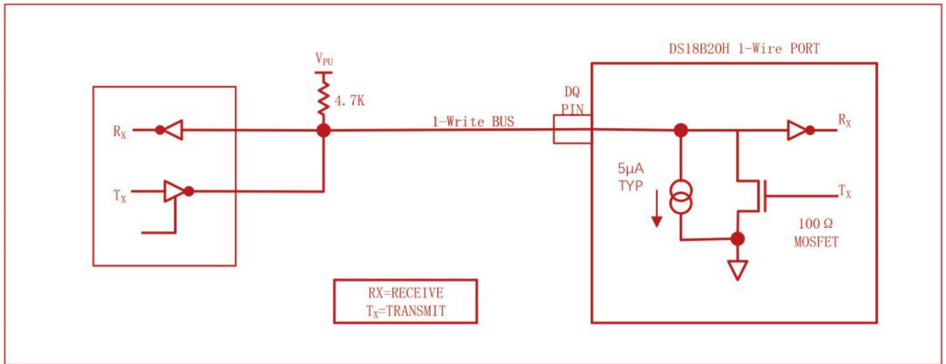
图 10. 硬件结构图
