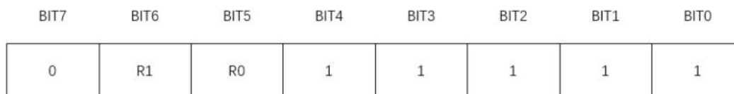
图 8. 配置寄存器
