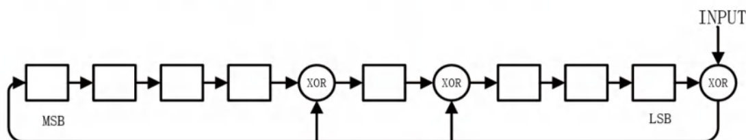
图 9. CRC 产生器
