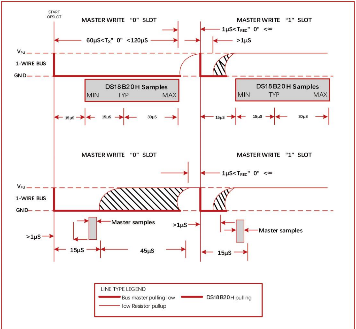
图 14. 读/写时序图
