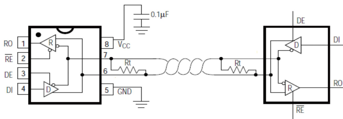
图1：MAX3485ESA典型半双工应用电路
