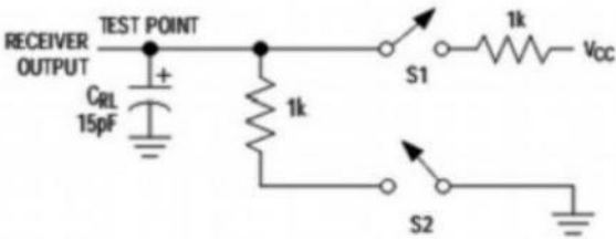
图4接收时间测试电路
