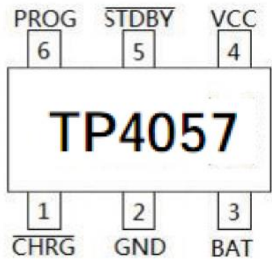
SOT-23-6L
