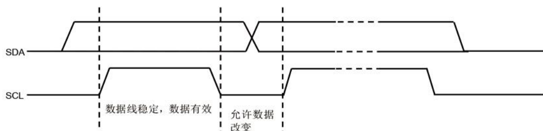
图 I 2 C 总线上的位传送
