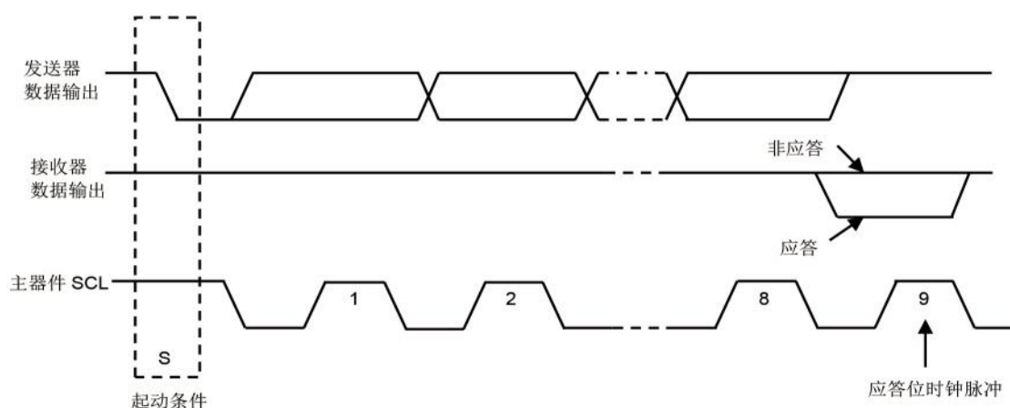
图 I 2 C 总线的应答位
