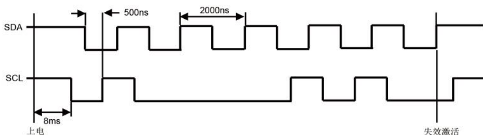
图 POR 失效时序图
