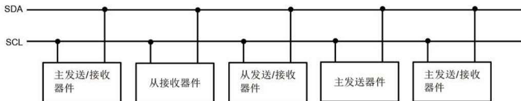
图 I 2 C 总线系统配置图
