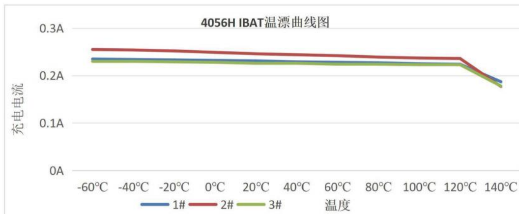
7.2 充电温漂曲线 (VIN=5V, PROG=5.1K)
