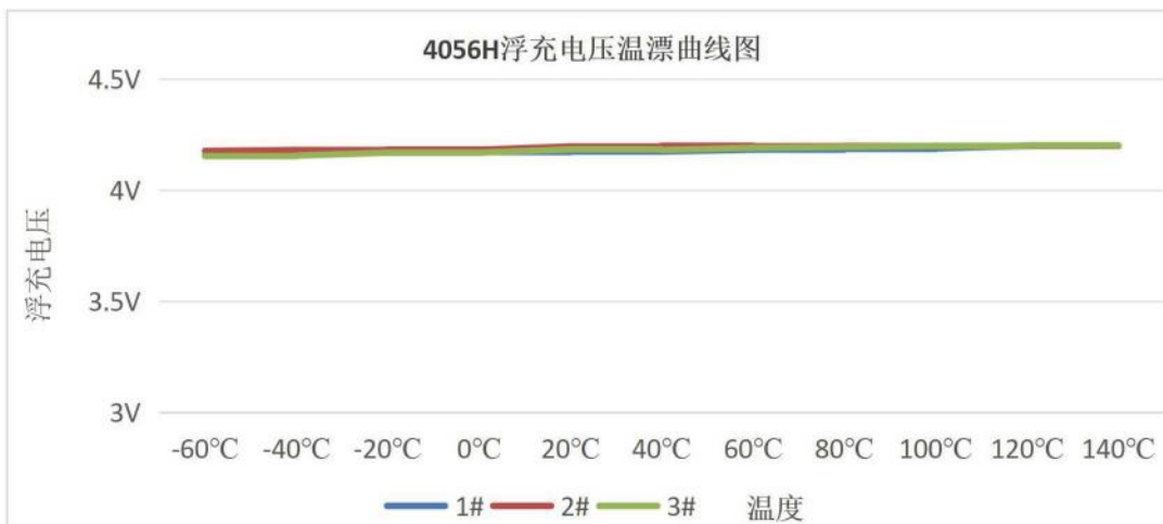
7.3 浮充电压温漂曲线 (VIN=5V, PROG=5.1K)
