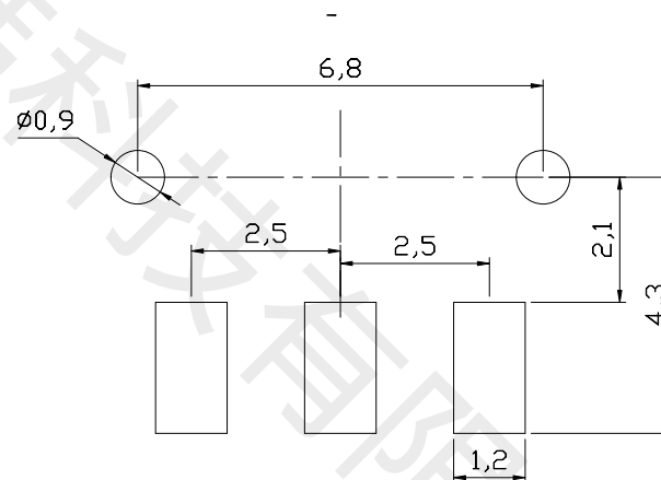
MSK12D 带柱
