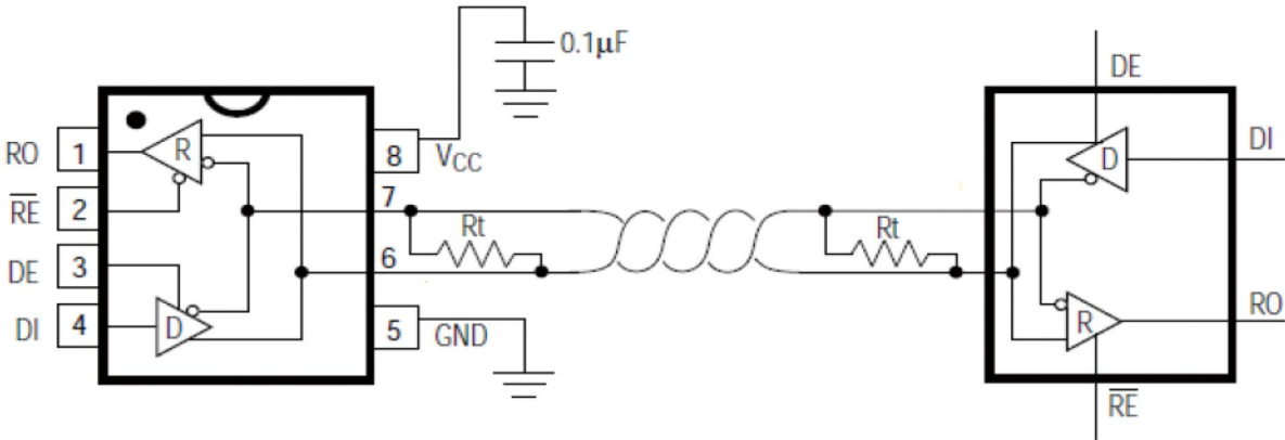
图1： SN65HVD3082DR-TD典型半双工应用电路
