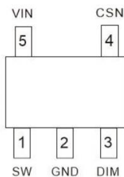
D3815C-TD(SOT23-5)
