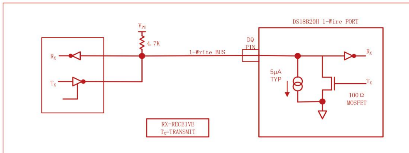
图 10. 硬件结构图
