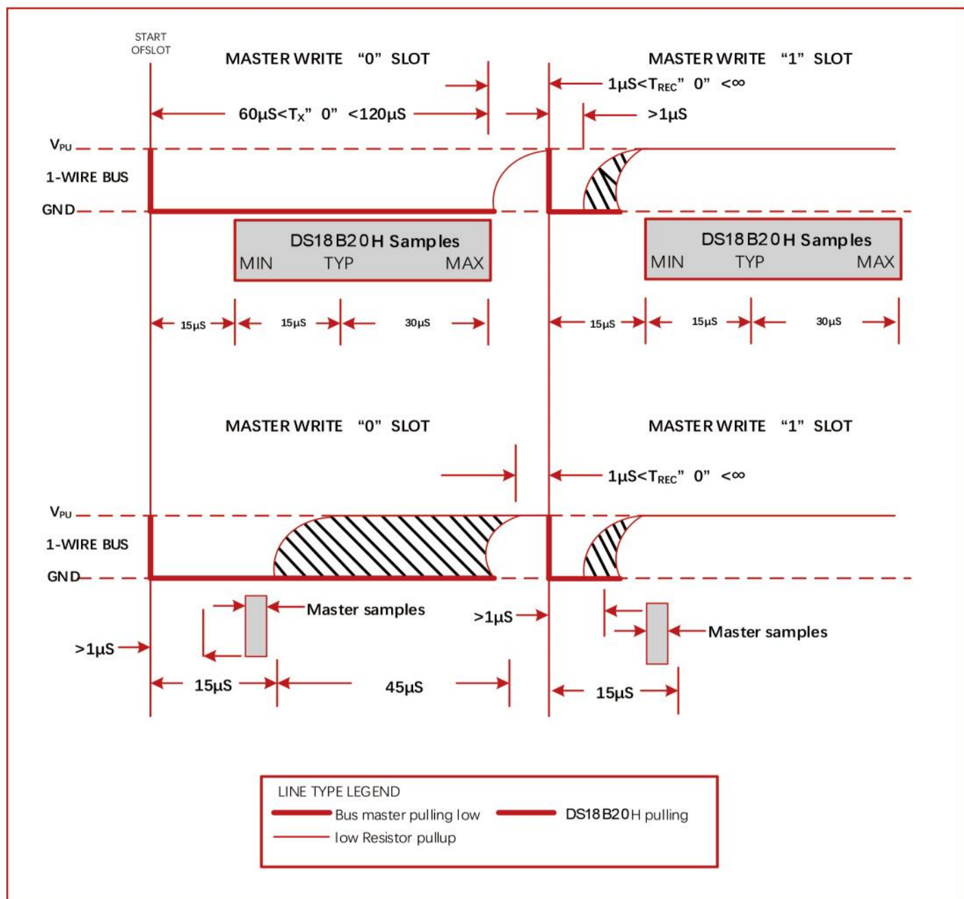
图 14. 读/写时序图
