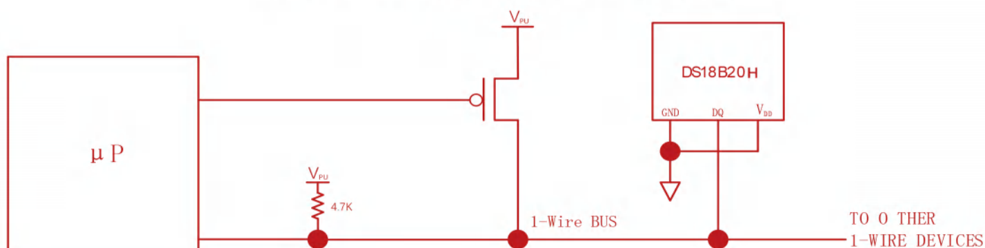
图 4. 在温度转换期间为寄生供电的 DS18B20供电
