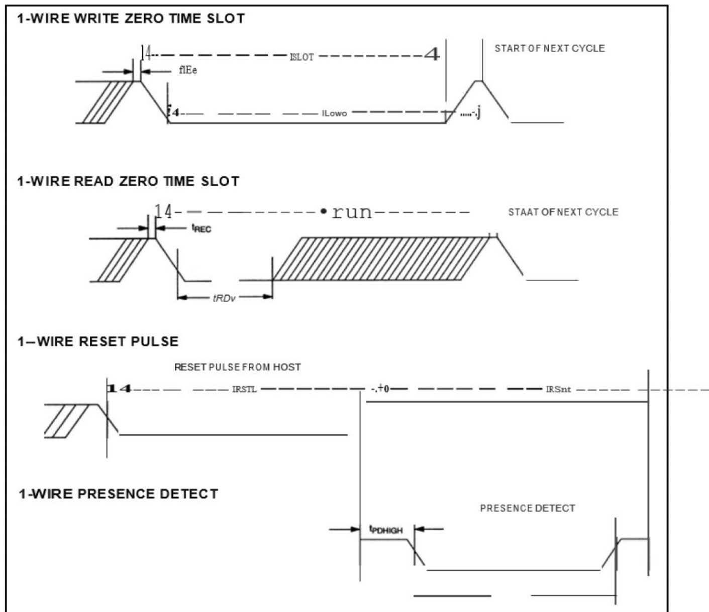
图 18. 时序
