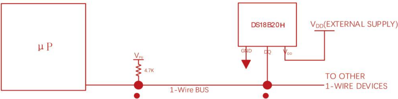
图 5. 使用外部电源为 DS18B20供电
