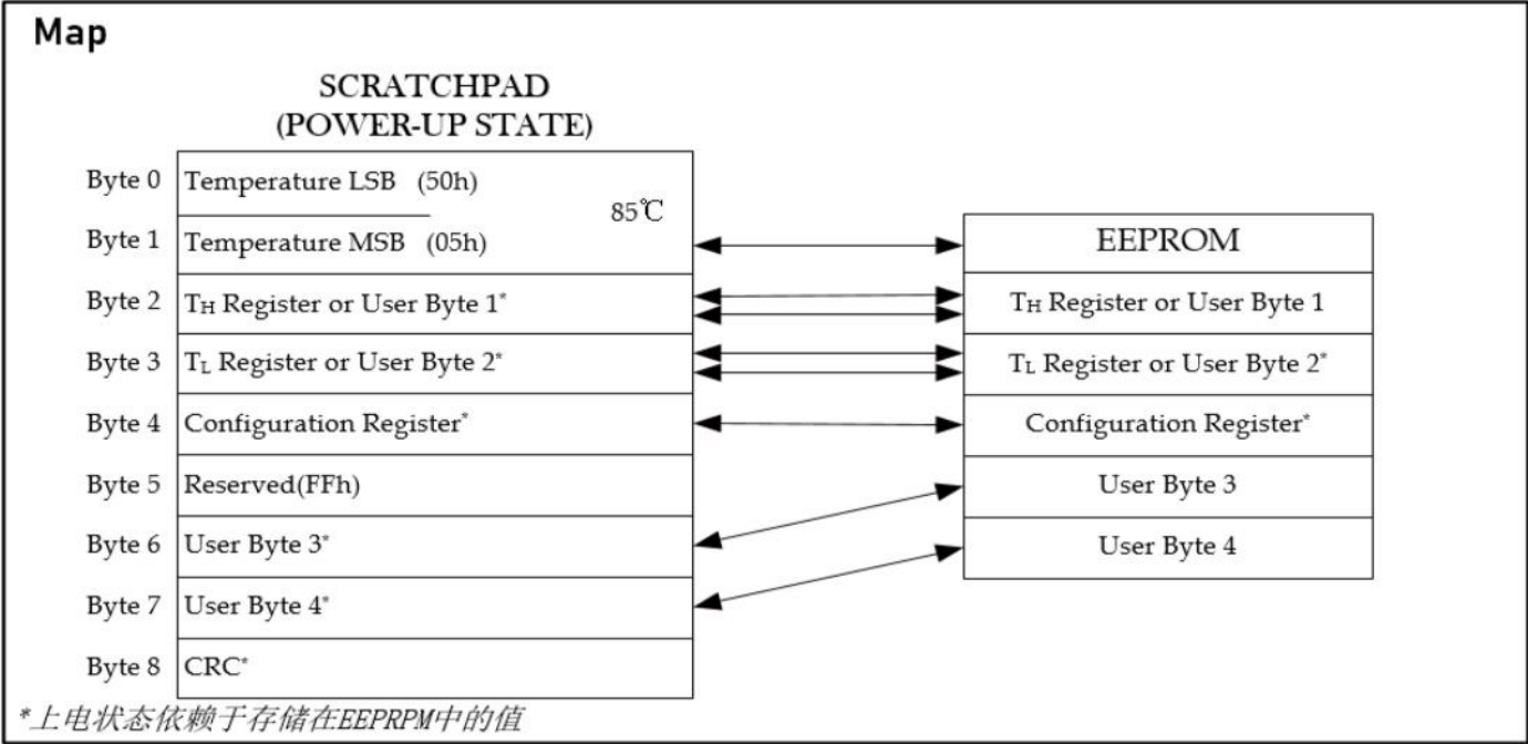
图 7. DS18B20存储器图
