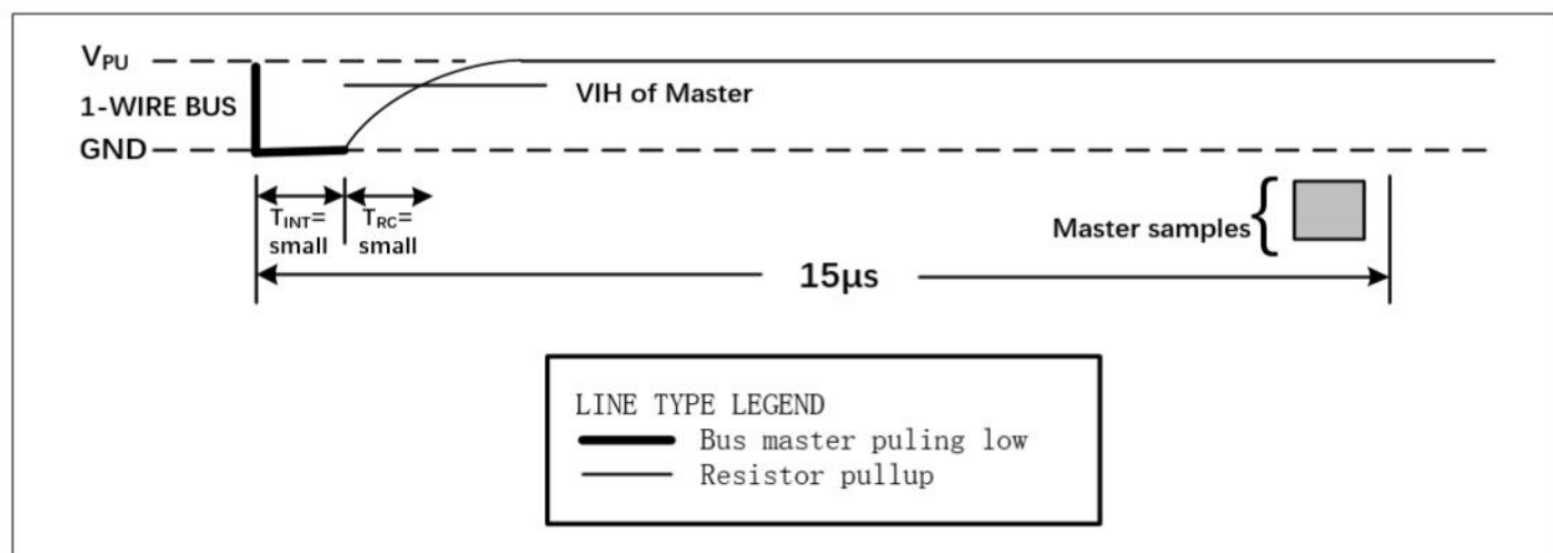
图 16. 推荐的控制读 1 时序
