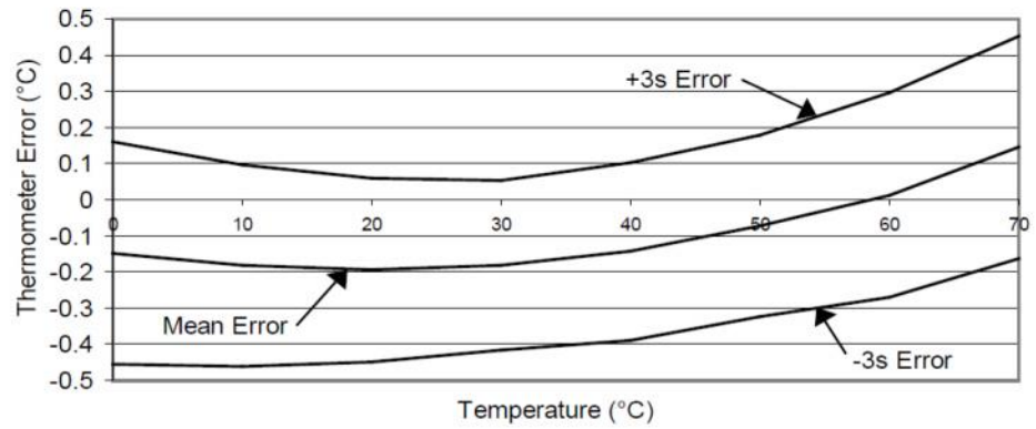
图 17. 典型的特性曲线
