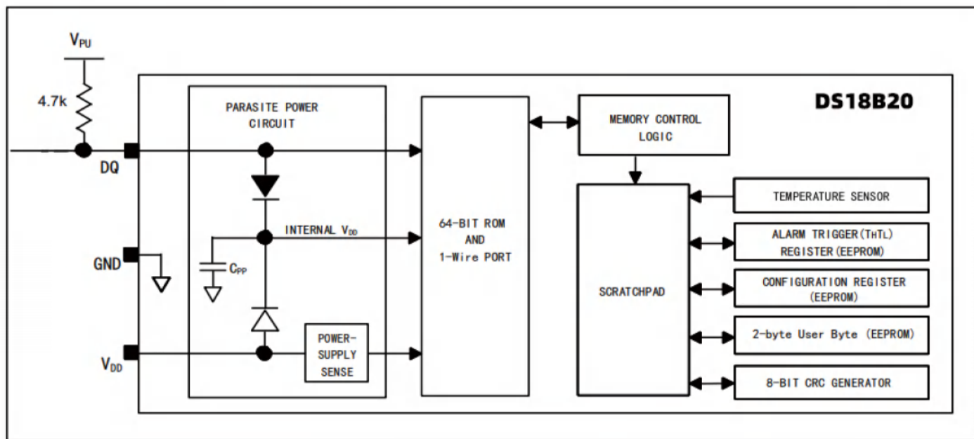
图 1. DS18B20结构框图
