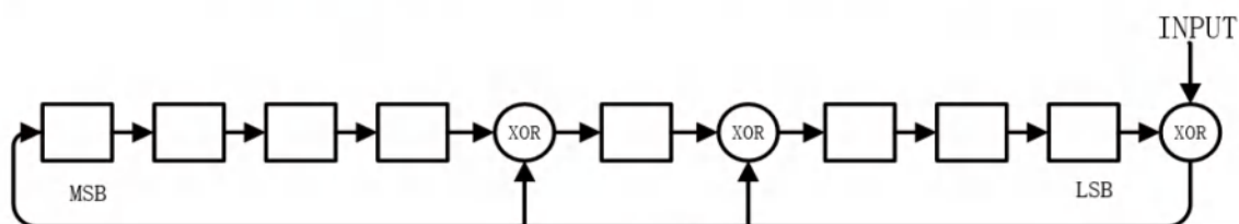
图 9. CRC 产生器
