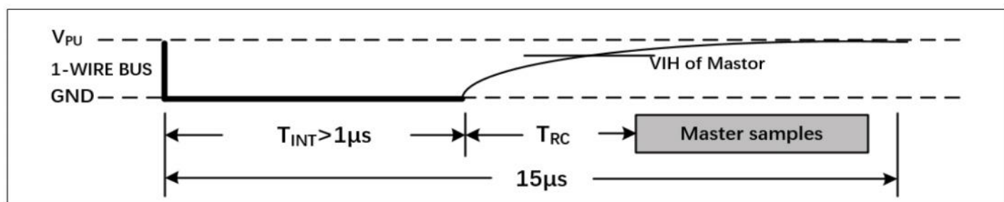
图 15. 控制器读 1 的详细时序
