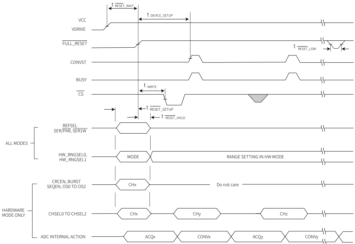
图 3 复位时序图
