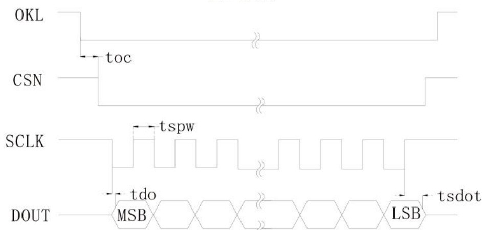
图 4 读时序
