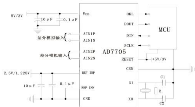
图 5 AD7705的电路图
