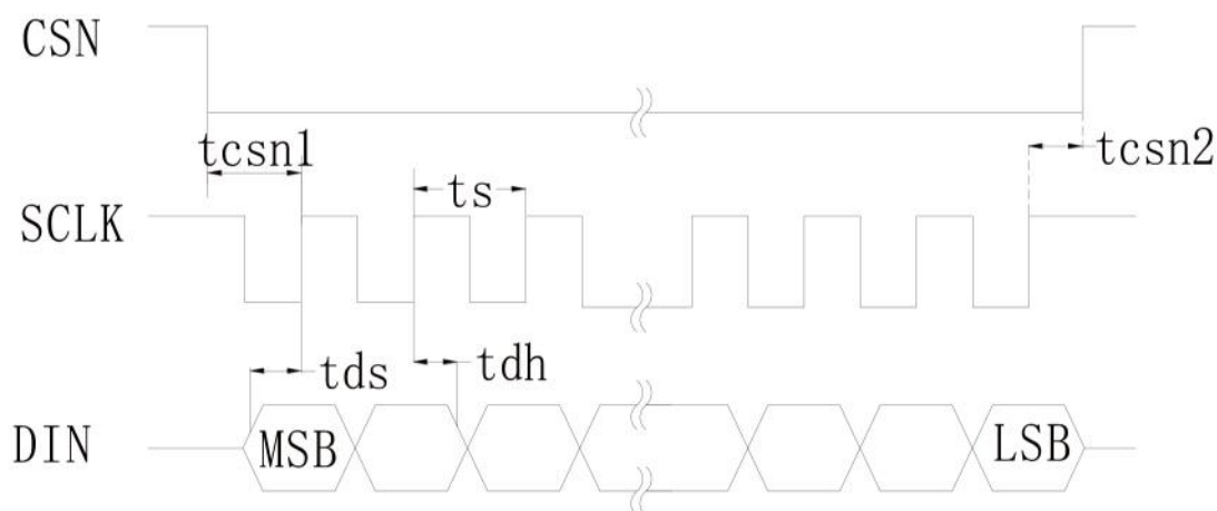
图 3 写时序
