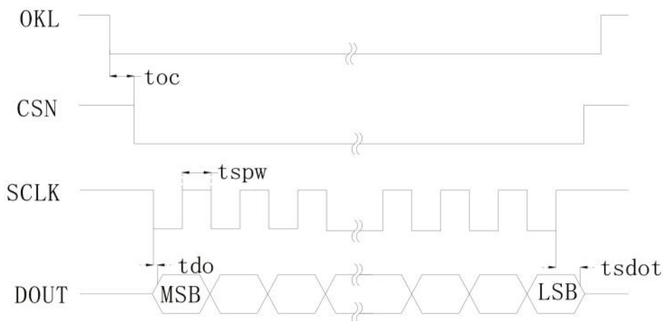
图 4 读时序
