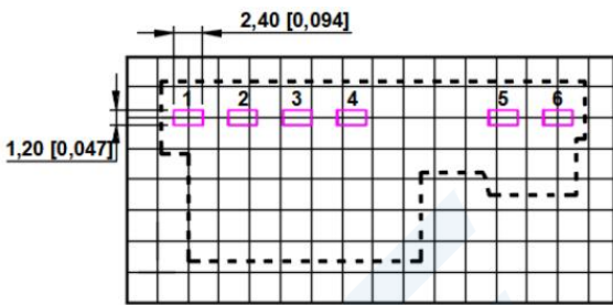
PCB 印刷版图
