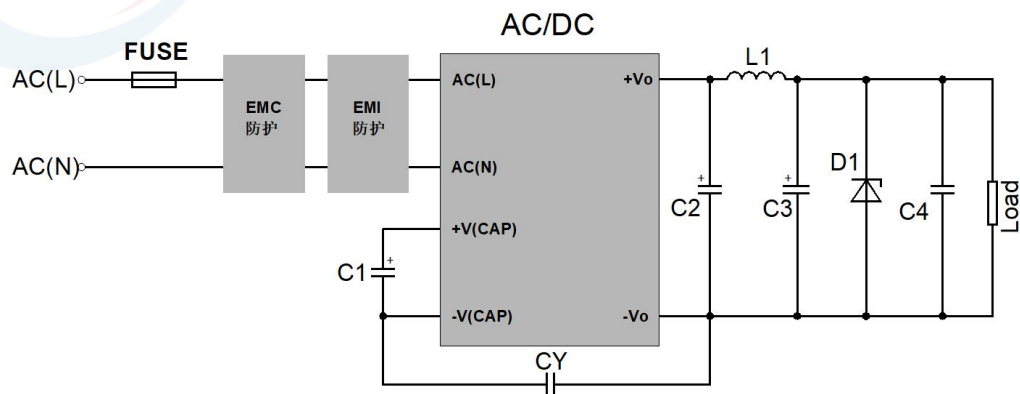
外围电路设计方案
