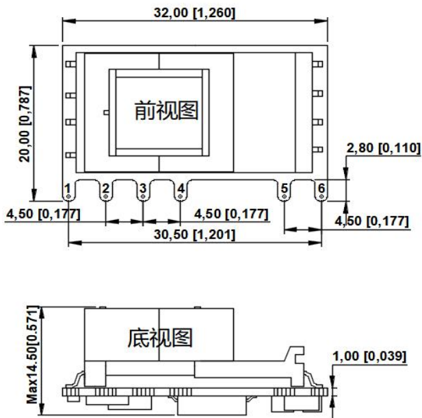
外观尺寸图
