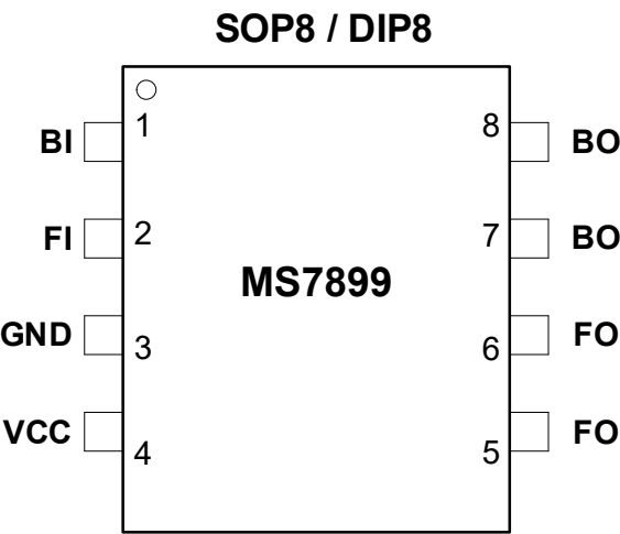
图 1. 顶视图
