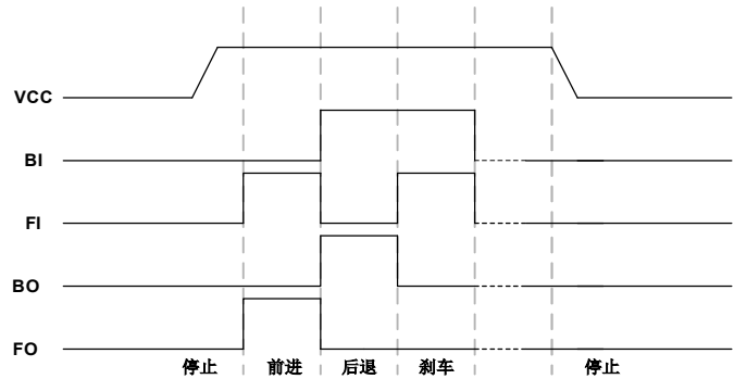
图 3. 输出时序图
