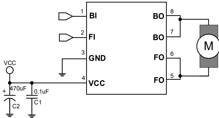
图 4. 应用原理图
