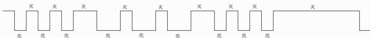
SOS波形图
