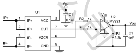
增益放大应用
