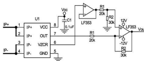
零点迁移应用
