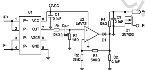
电流峰值监测应用
