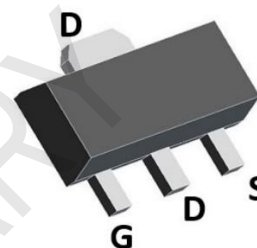
SOT-89
